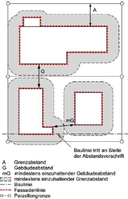
Figur 6.1–6.3 Abstände und Abstandsbereiche
