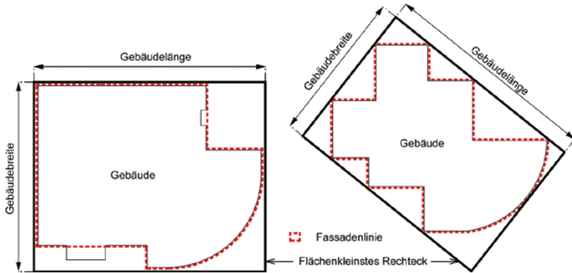
Figur 3.1 und 3.2 Gebäuelänge und Gebäudebreite
